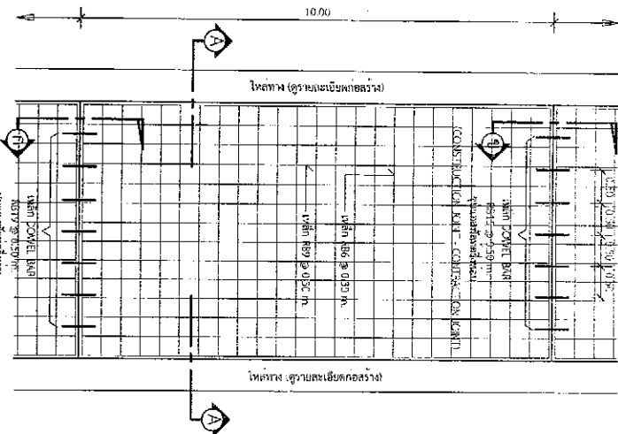
แบบถนนถนน 1 : 75
