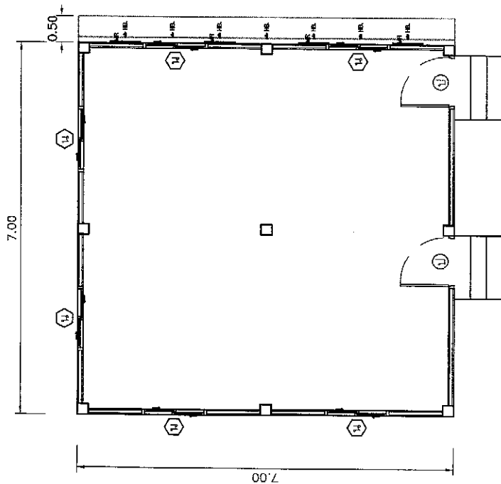
แปลนใหม่ NOSCALE
